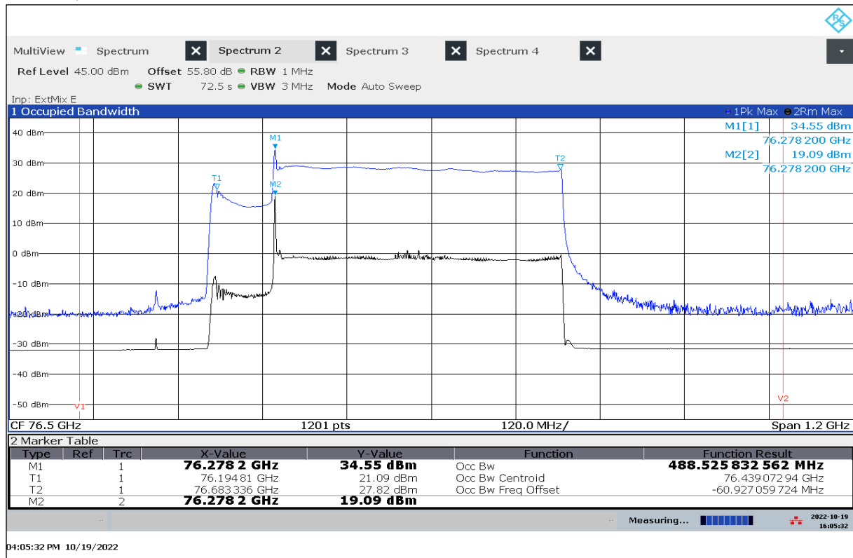
Plot 22: OBW, 0 °C / V nom
