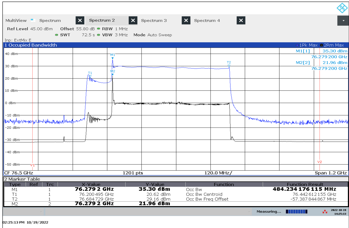
Plot 19: OBW, T_{\min} / V_{\text{nom}}
