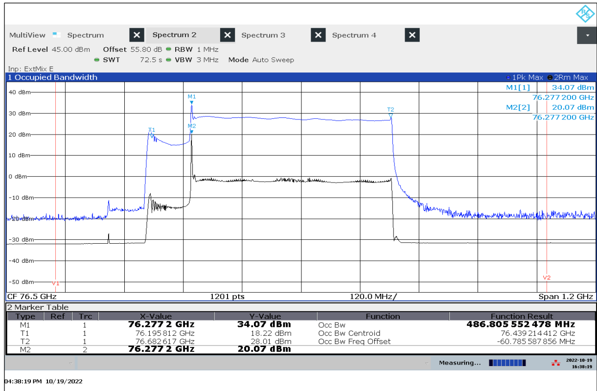
Plot 23: OBW, +10 °C / V nom
