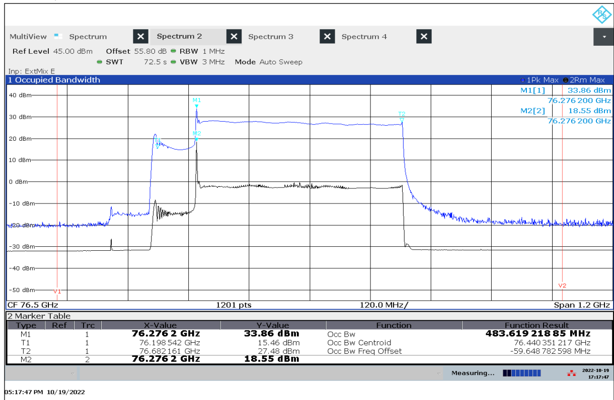
Plot 24: OBW, +20 °C / V nom
