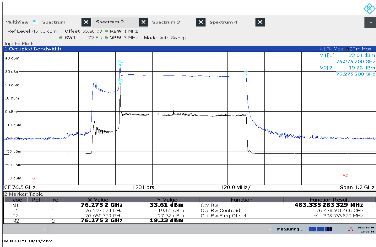
Plot 27: OBW, +50 °C / V nom
