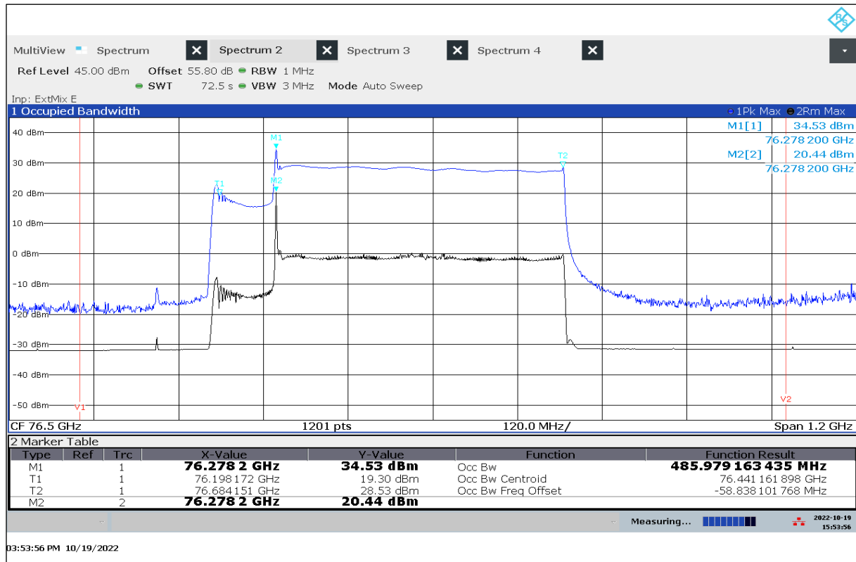
Plot 21: OBW, -10 °C / V nom
