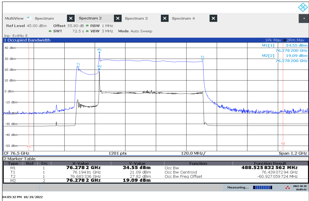
Plot 20: OBW, -20 °C / V_{\text{nom}}
