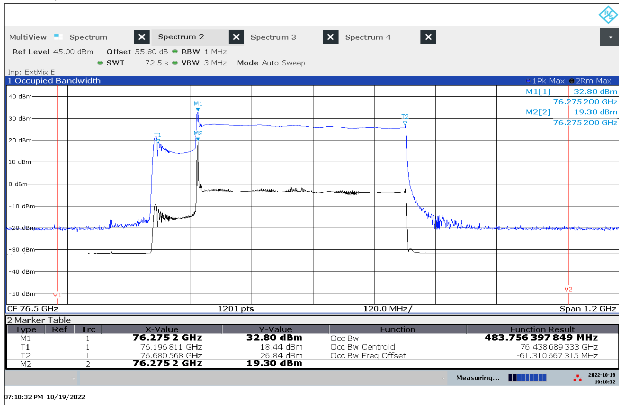
Plot 28: OBW, T max / V nom
