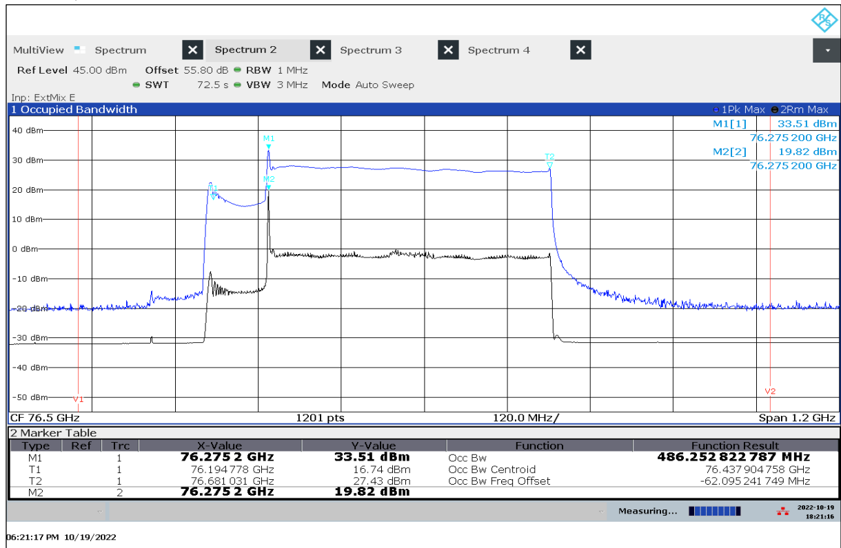
Plot 26: OBW, +40 °C / V_{nom}
