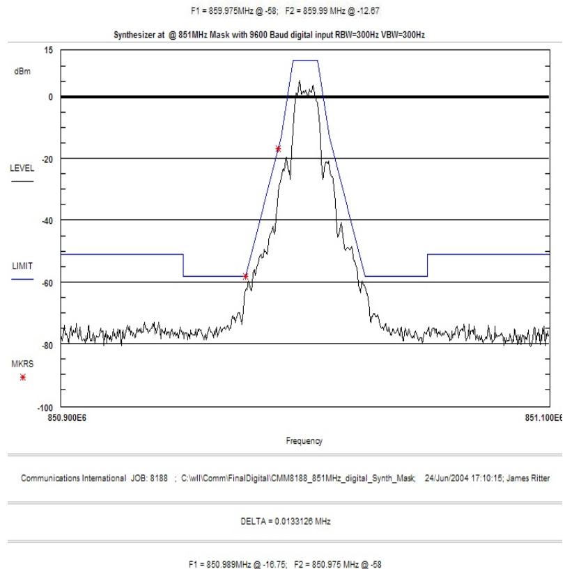
Figure 12. Mask, 851 MHz Digital Modulation F1D, F1E, F2D, F2B
