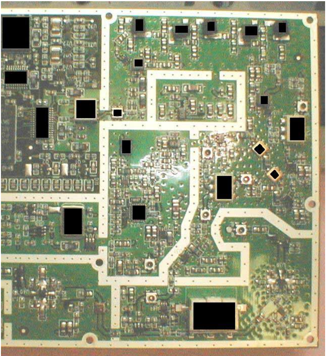
PCB Bottom
