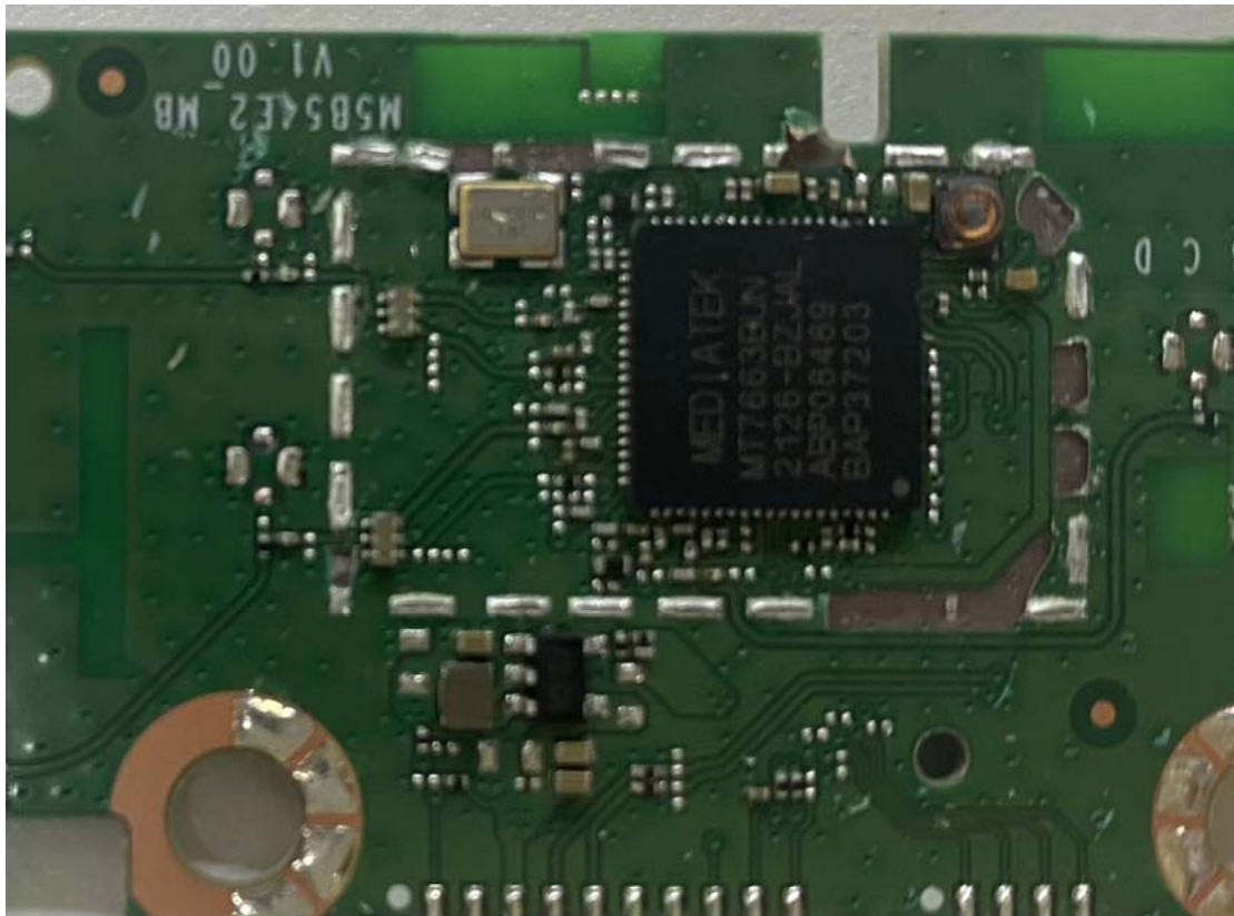
IC details
