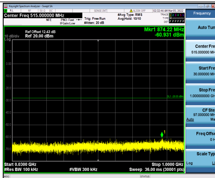
11AC40SISO_Ant2_2422_30~1000
