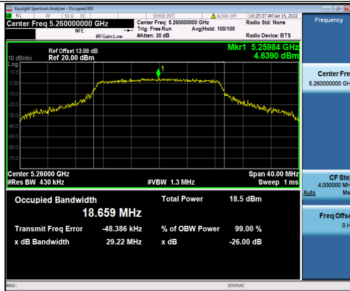
11N20MIMO_Ant2_5260
