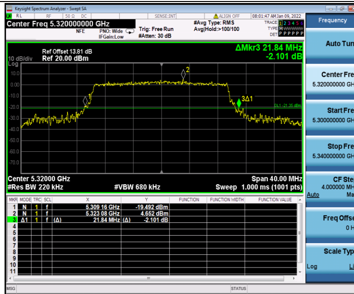
11AX20SISO_Ant2_5320
