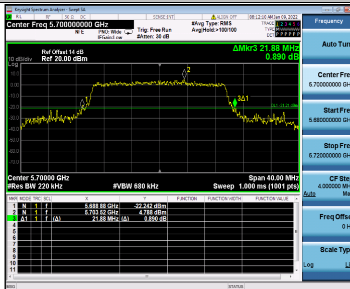
11AX20SISO_Ant2_5700
