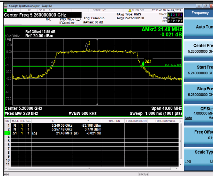
11AX20SISO_Ant2_5260
