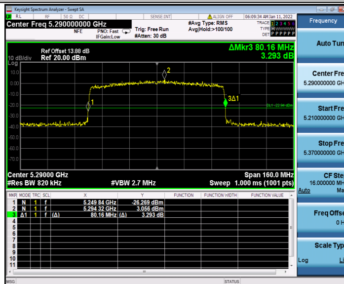
11AX80SISO_Ant2_5290
