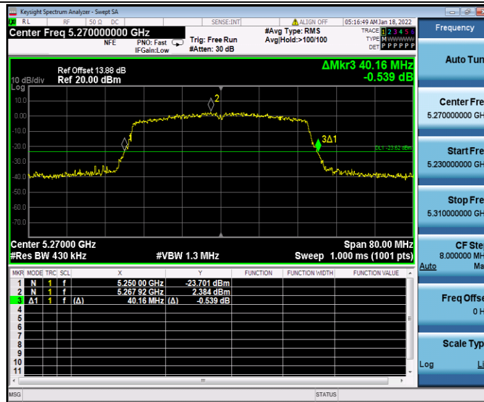
11AC40MIMO_Ant2_5270
