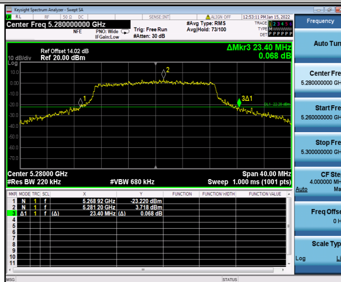
11AC20MIMO_Ant2_5280
