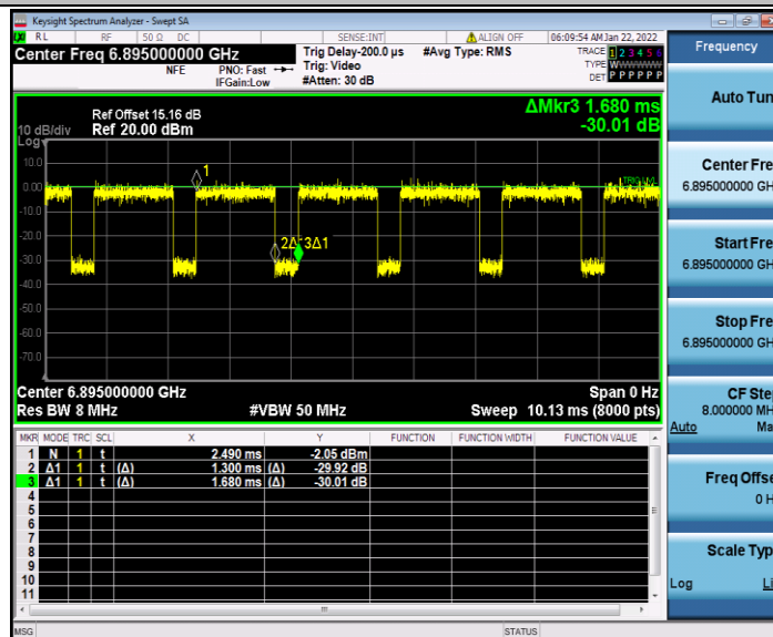
11N20SISO_Ant2_6895
