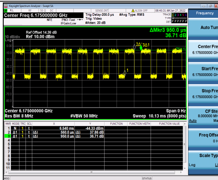
11AX20MIMO_Ant2_6175
