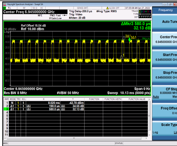
11AC80MIMO_Ant2_6945
