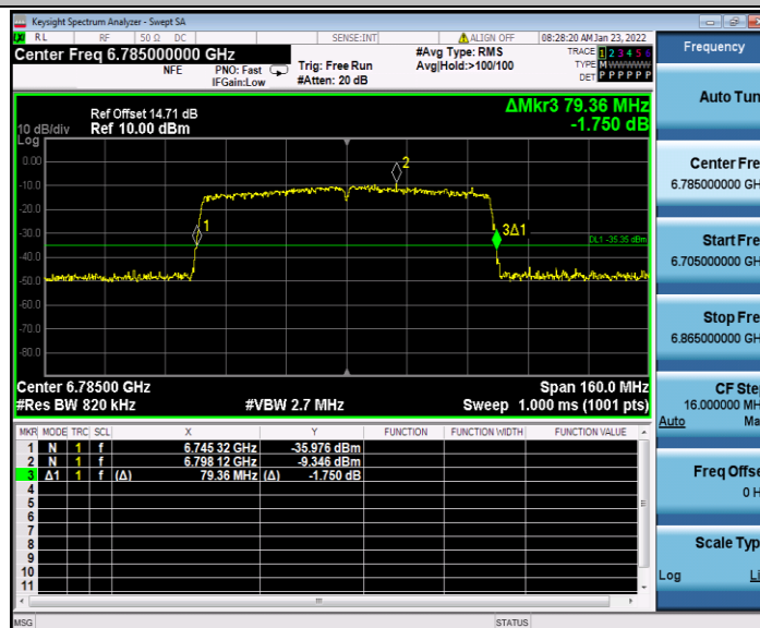
11AC80SISO_Ant1_6785
