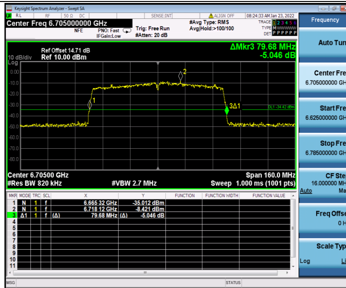
11AC80SISO_Ant2_6705
