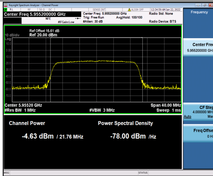
11AX20SISO_Ant2_5955
