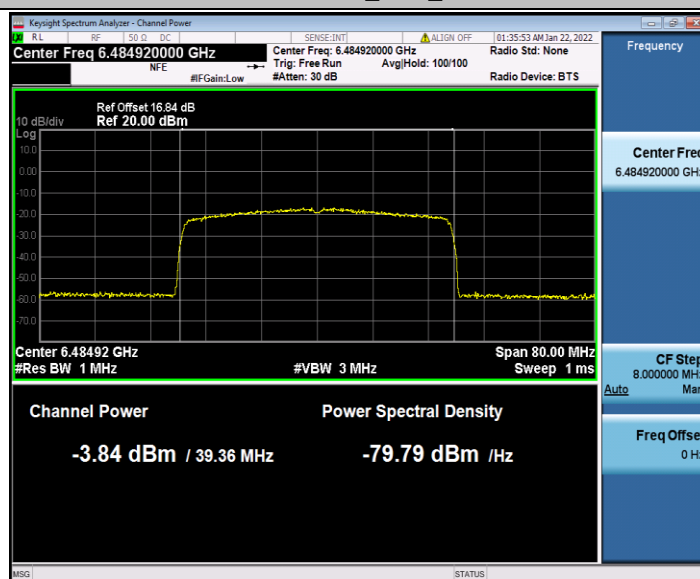
11AX40SISO_Ant1_6485
