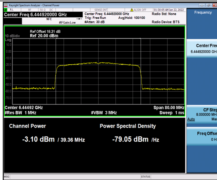
11AX40SISO_Ant2_6445
