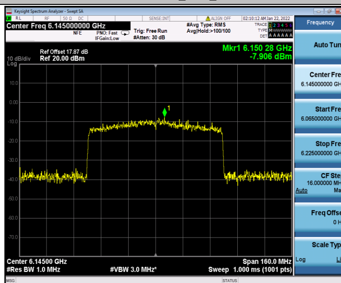
11AX80SISO_Ant1_6145
