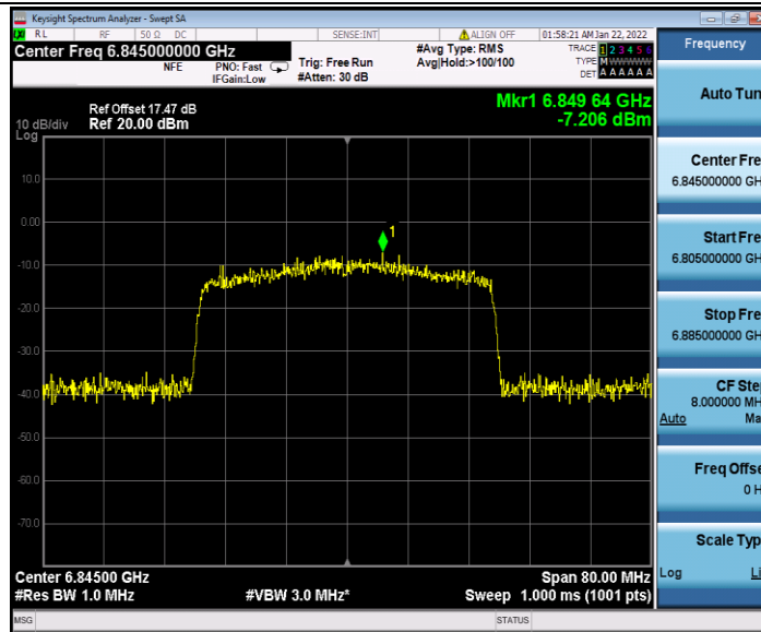
11AX40SISO_Ant2_6845
