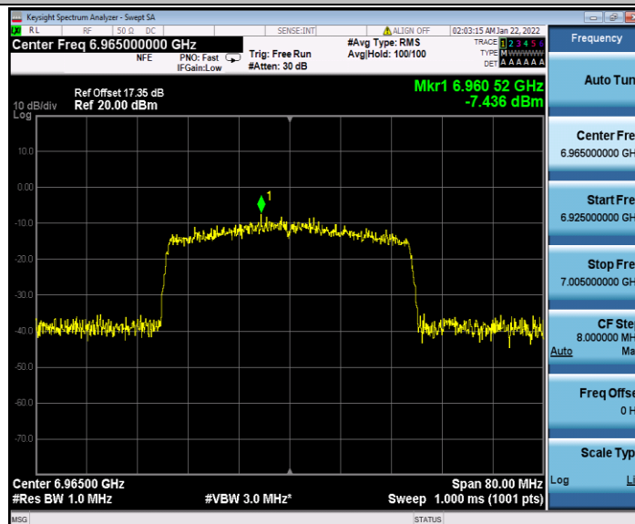
11AX40SISO_Ant2_6965
