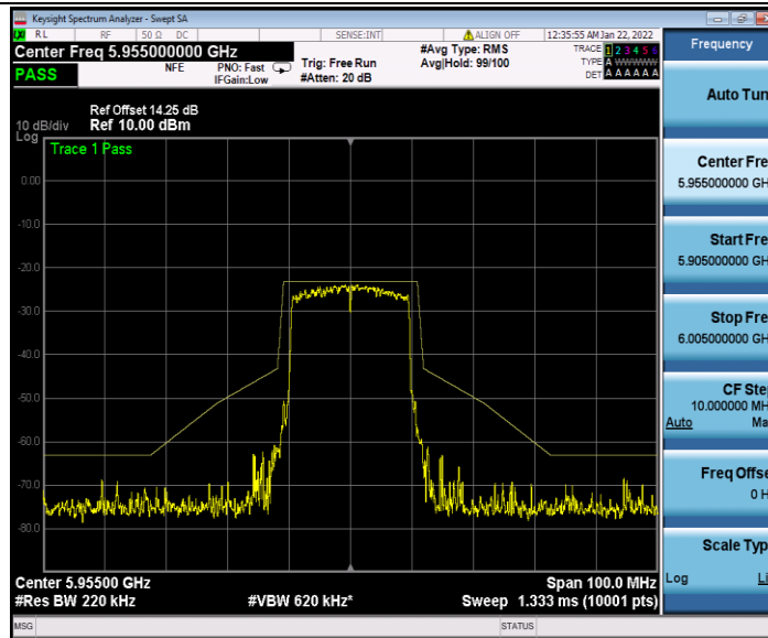
11AX20SISO_Ant2_5955
