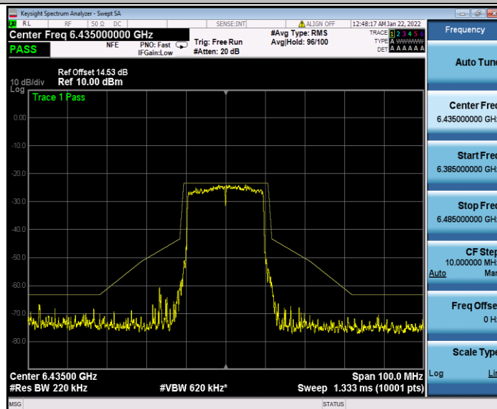
11AX20SISO_Ant2_6435
