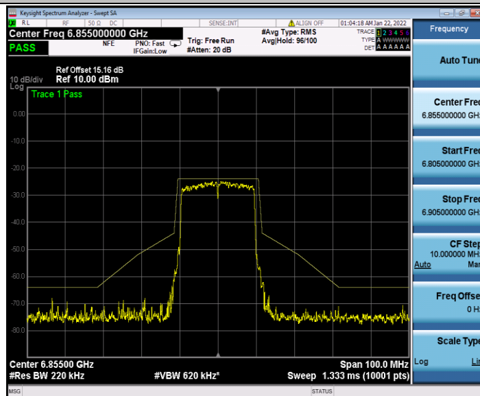
11AX20SISO_Ant2_6855
