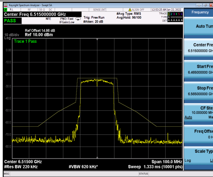
11AX20SISO_Ant2_6515
