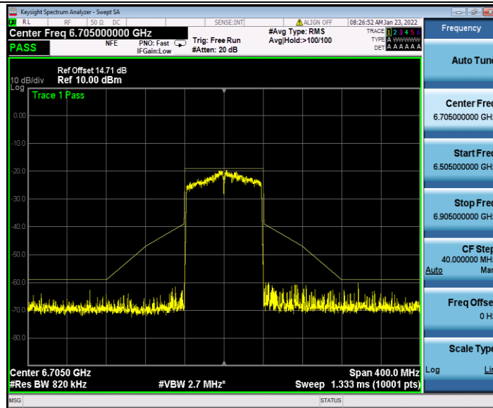
11AC80SISO_Ant2_6705
