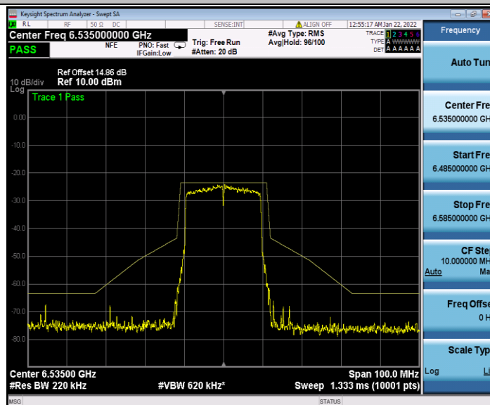
11AX20SISO_Ant1_6535
