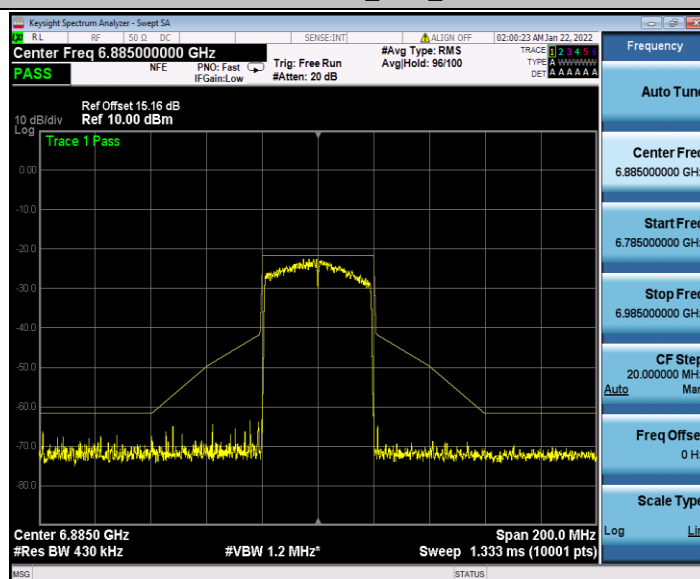
11AX40SISO_Ant1_6885
