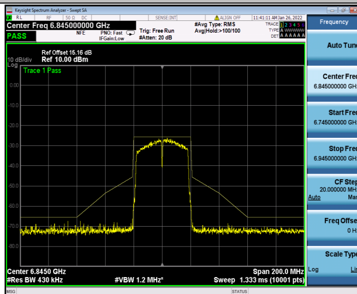
11AC40MIMO_Ant1_6845
