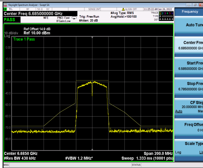
11AC40MIMO_Ant2_6685
