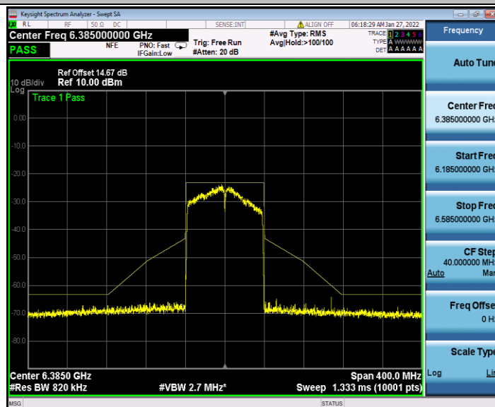
11AC80MIMO_Ant2_6385
