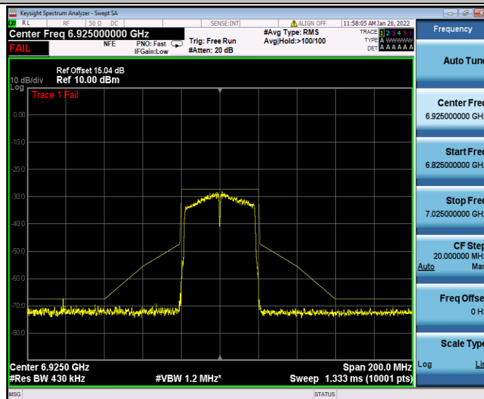
11AC40MIMO_Ant2_6925
