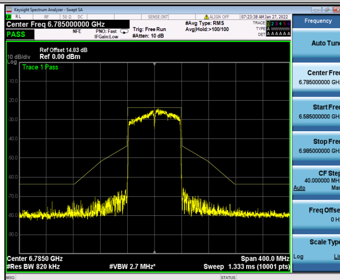
11AC80MIMO_Ant2_6785
