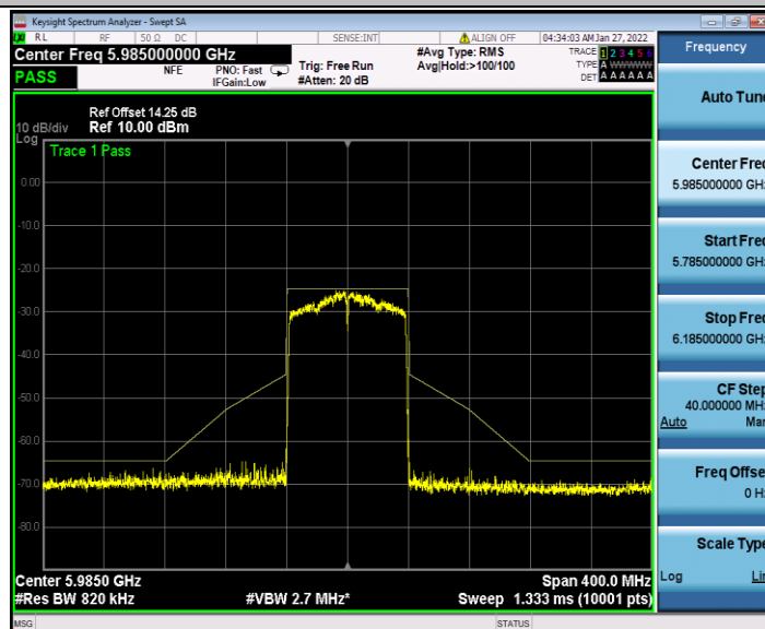
11AC80MIMO_Ant1_5985
