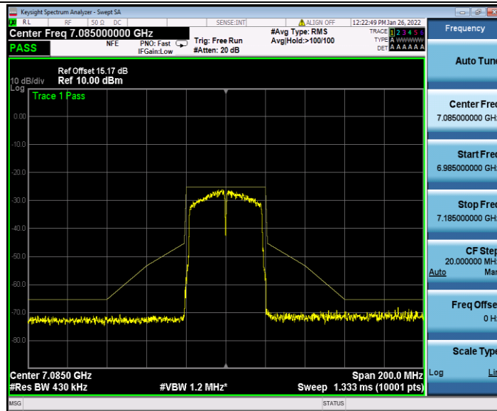
11AC40MIMO_Ant2_7085
