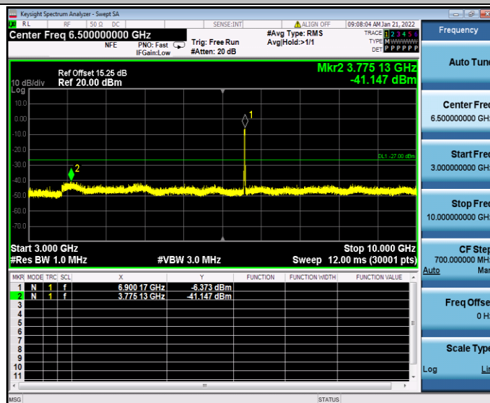
11AX20SISO_Ant2_6895_3000~10000
