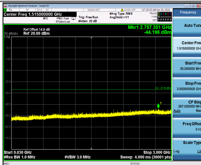
11N20MIMO_Ant1_6695_30~3000
