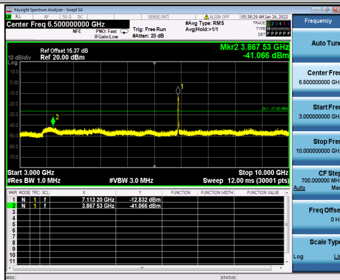
11AC20MIMO_Ant1_7115_3000~10000
