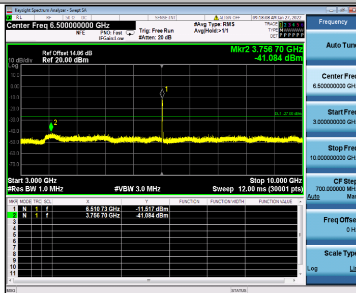
11AX20MIMO_Ant1_6515_3000~10000
