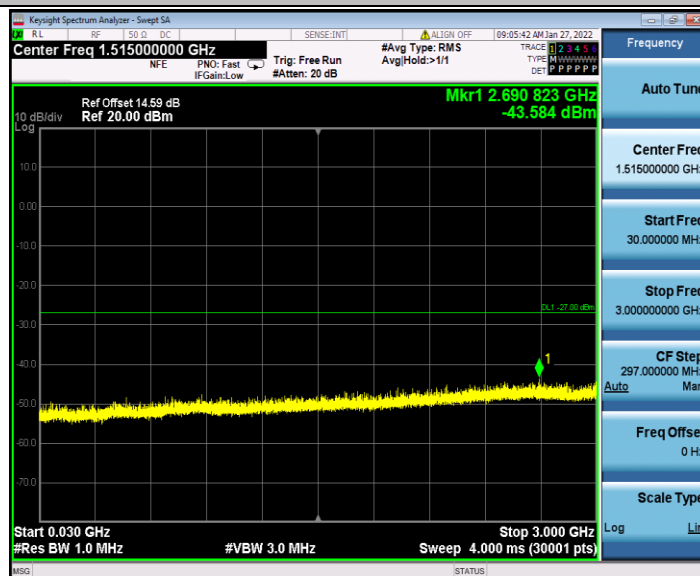
11AX20MIMO_Ant2_6435_30~3000
