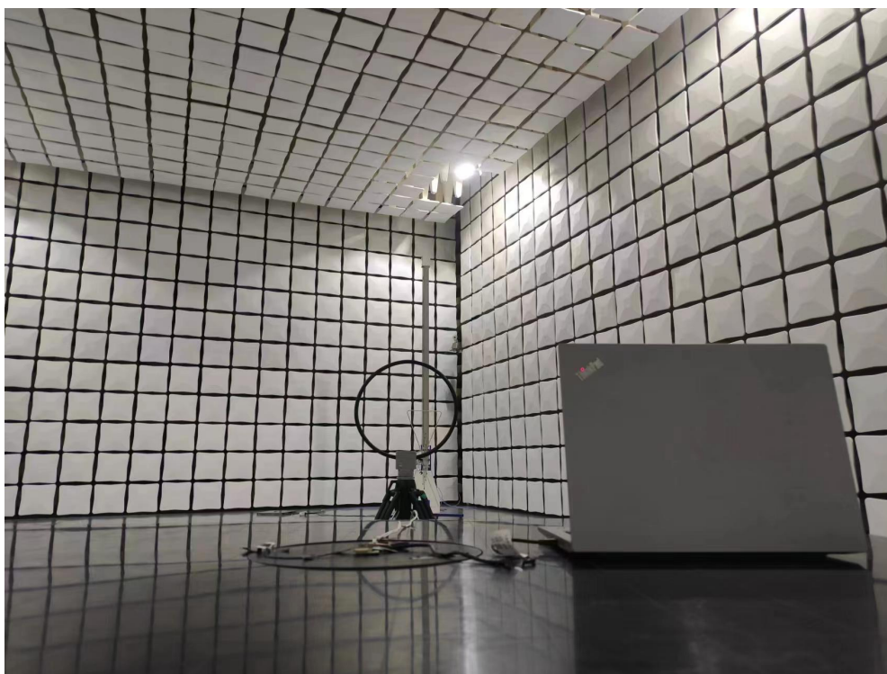
9KHz~30MHz
