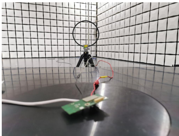
9KHz~30MHz
