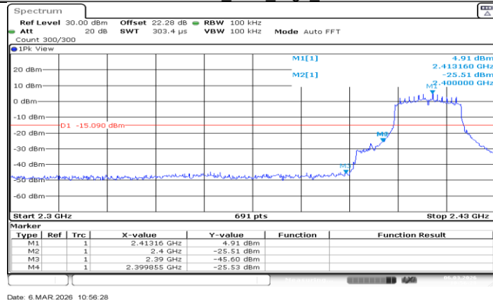
11N20MIMO_Ant1_Low_2412
