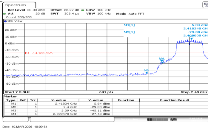
11G-CDD_Ant2_Low_2417
