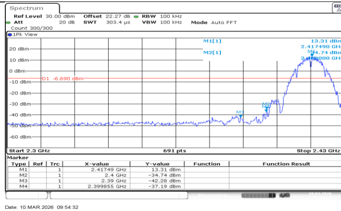
11B-CDD_Ant2_Low_2417
