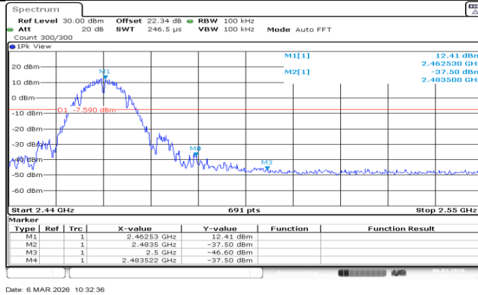
11B-CDD_Ant1_High_2462
