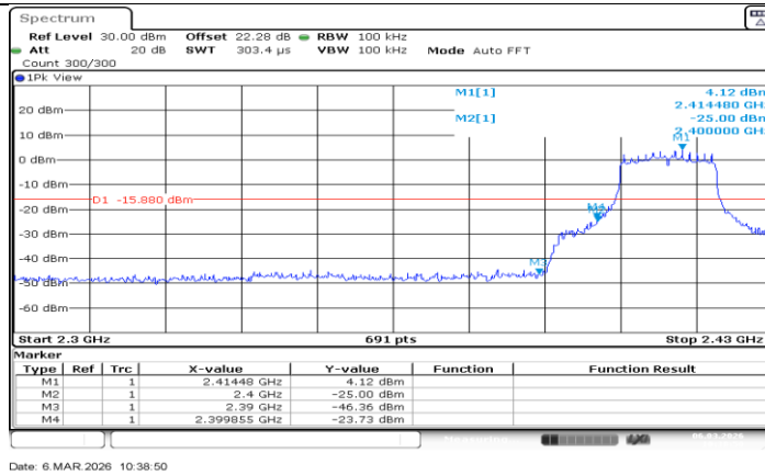
11G-CDD_Ant1_Low_2412
