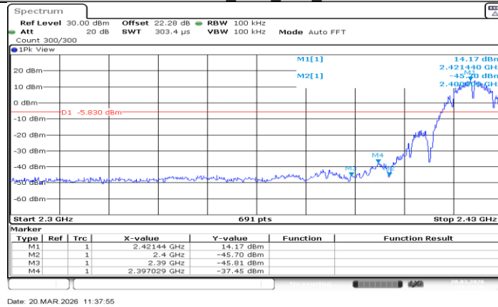
11B-CDD_Ant1_Low_2422
