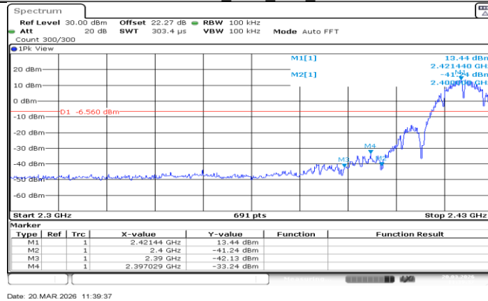
11B-CDD_Ant2_Low_2422
