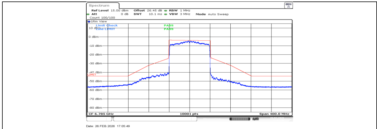
11AX80MIMO_Ant4_6785
