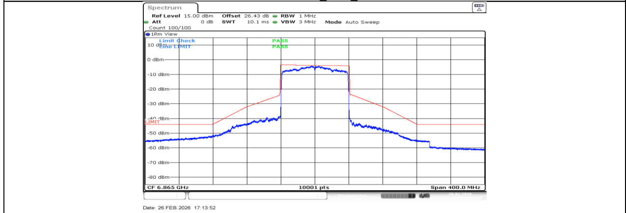
11AX80MIMO_Ant4_6865
