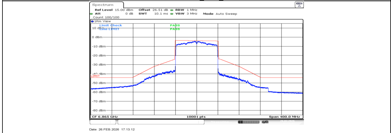
11AX80MIMO_Ant3_6865
