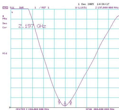
(측정지그에서 측정)
