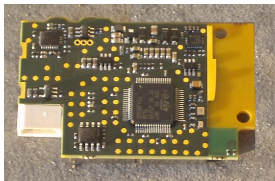
PCB bottom
