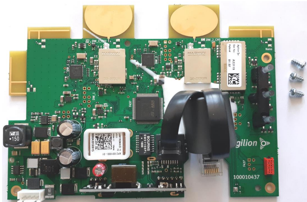
PCB top
