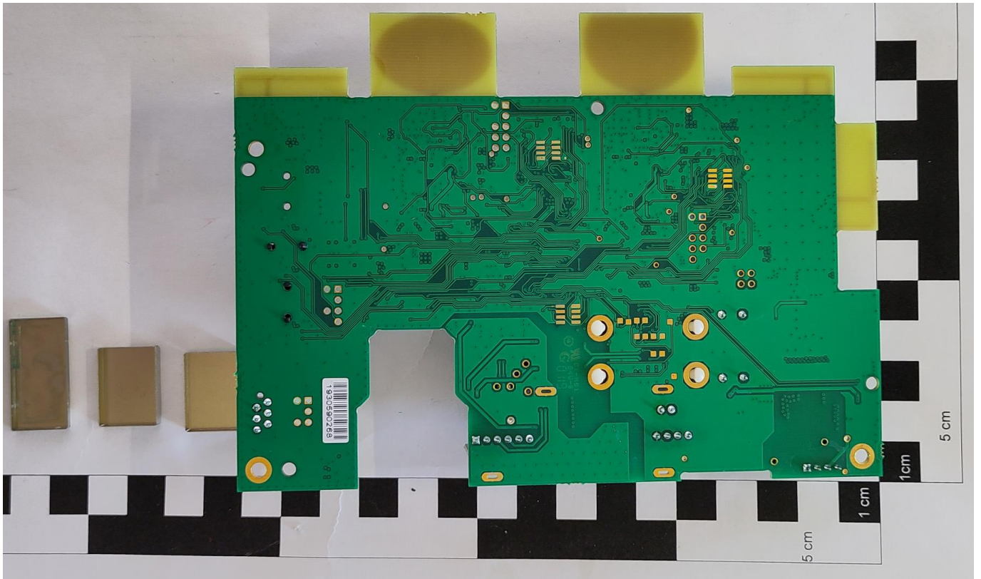
PCB bottom
