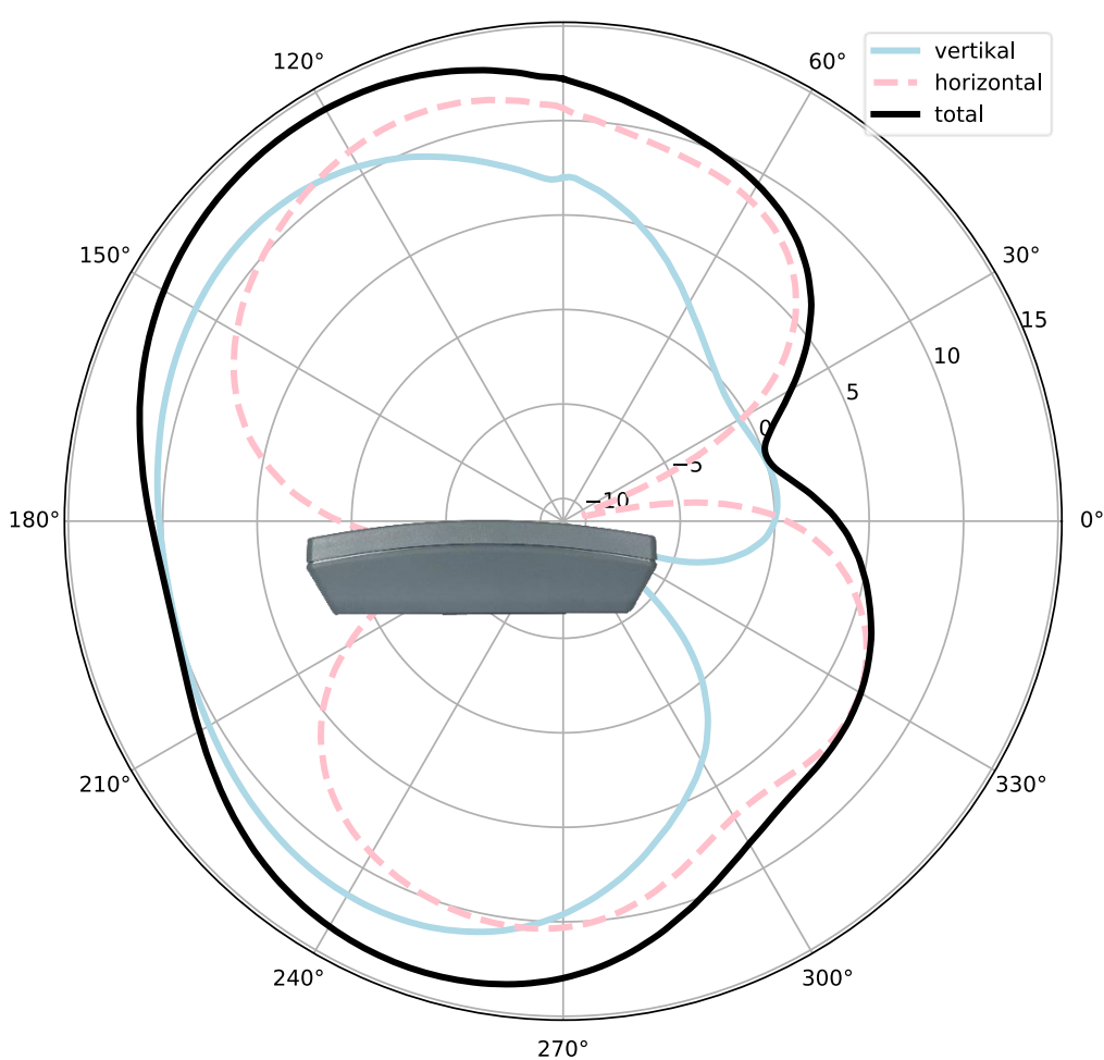
EIRP/dBm 2,4GHz 3 / IF1, azimuthal, Frontdeckel bei 90°
