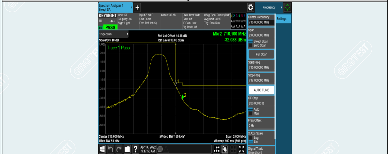
Band12-3MHz-QPSK-23165-1RB#14
