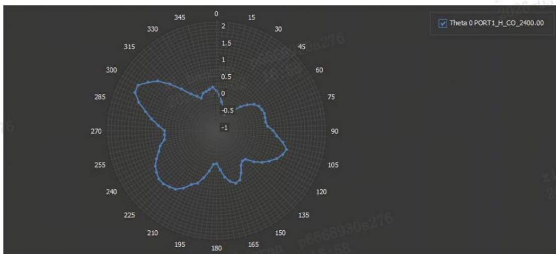
图 1: 1#样品 (2D 辐射方向图, 2400.00MHz, \Theta=0^\circ )
