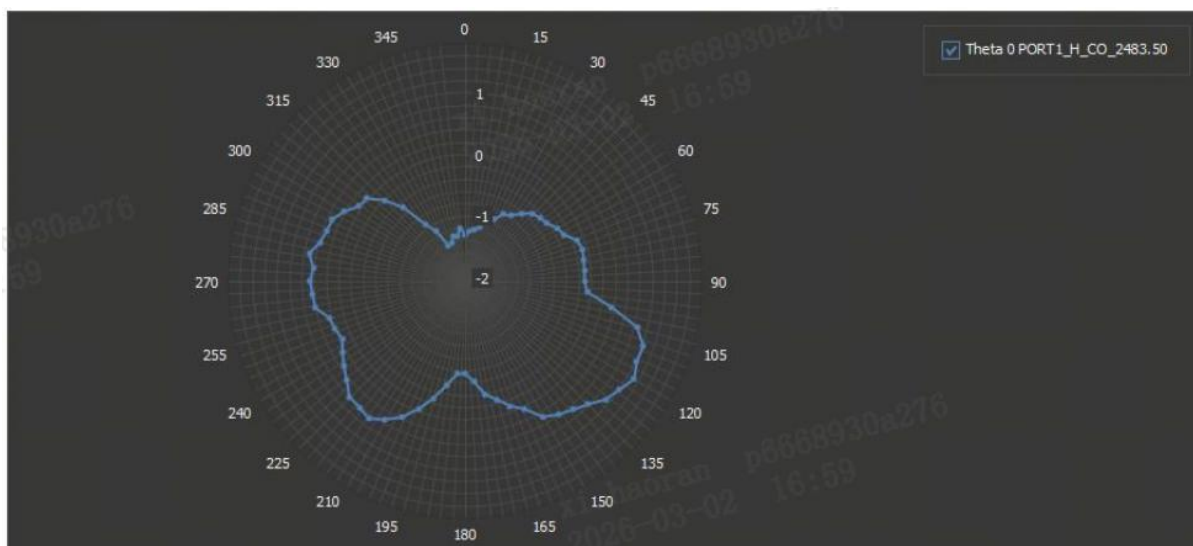
图 5: 1#样品 (2D 辐射方向图, 2483.50MHz, \Theta=0^\circ )
