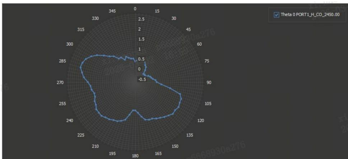
图 3: 1#样品 (2D 辐射方向图, 2450.00MHz, Theta=0° )
