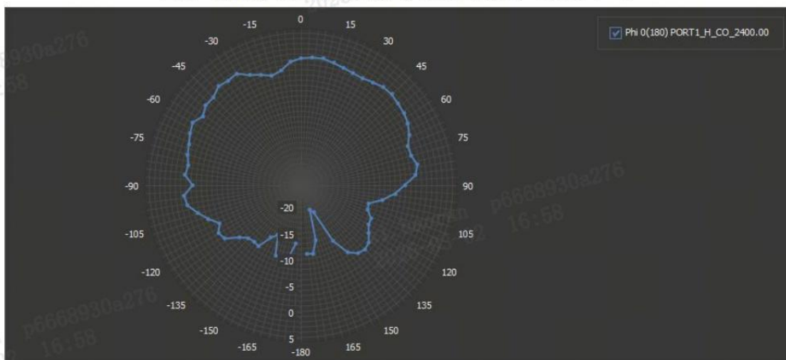
图 2: 1#样品 (2D 辐射方向图, 2400.00MHz, \Phi=0^\circ/180^\circ )
