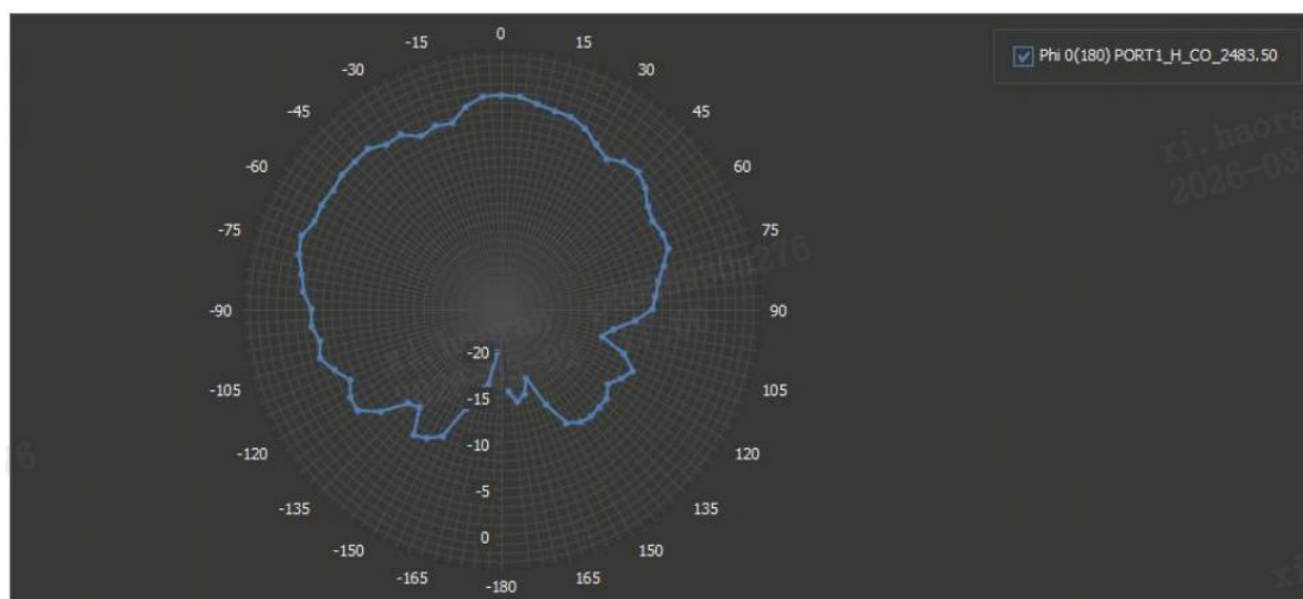
图 6: 1#样品 (2D 辐射方向图, 2483.50MHz, \Phi=0^\circ / 180^\circ )
