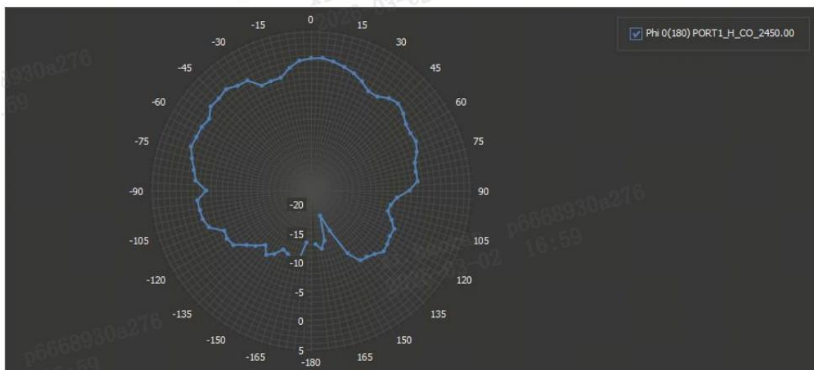
图 4: 1#样品 (2D 辐射方向图, 2450.00MHz, Phi=0° /180° )
