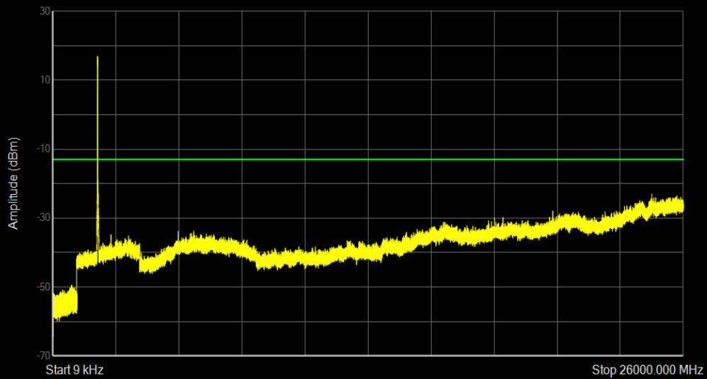
Band2 16QAM BW=20MHz Channel=18700 RB Size=100 Position=#0
