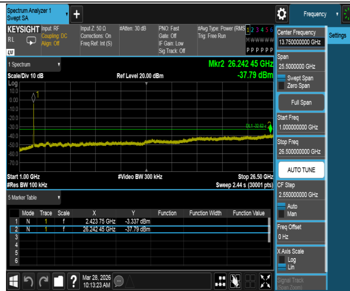
11N40MIMO_Ant0_2437_0~Reference
