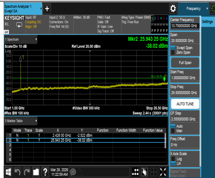
11AX40MIMO_Ant1_2422_0~Reference
