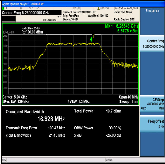
11A-Ant1-5260
