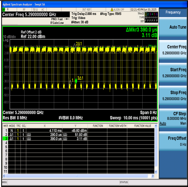
NTNV-11AX80SISO-Ant1-5290
