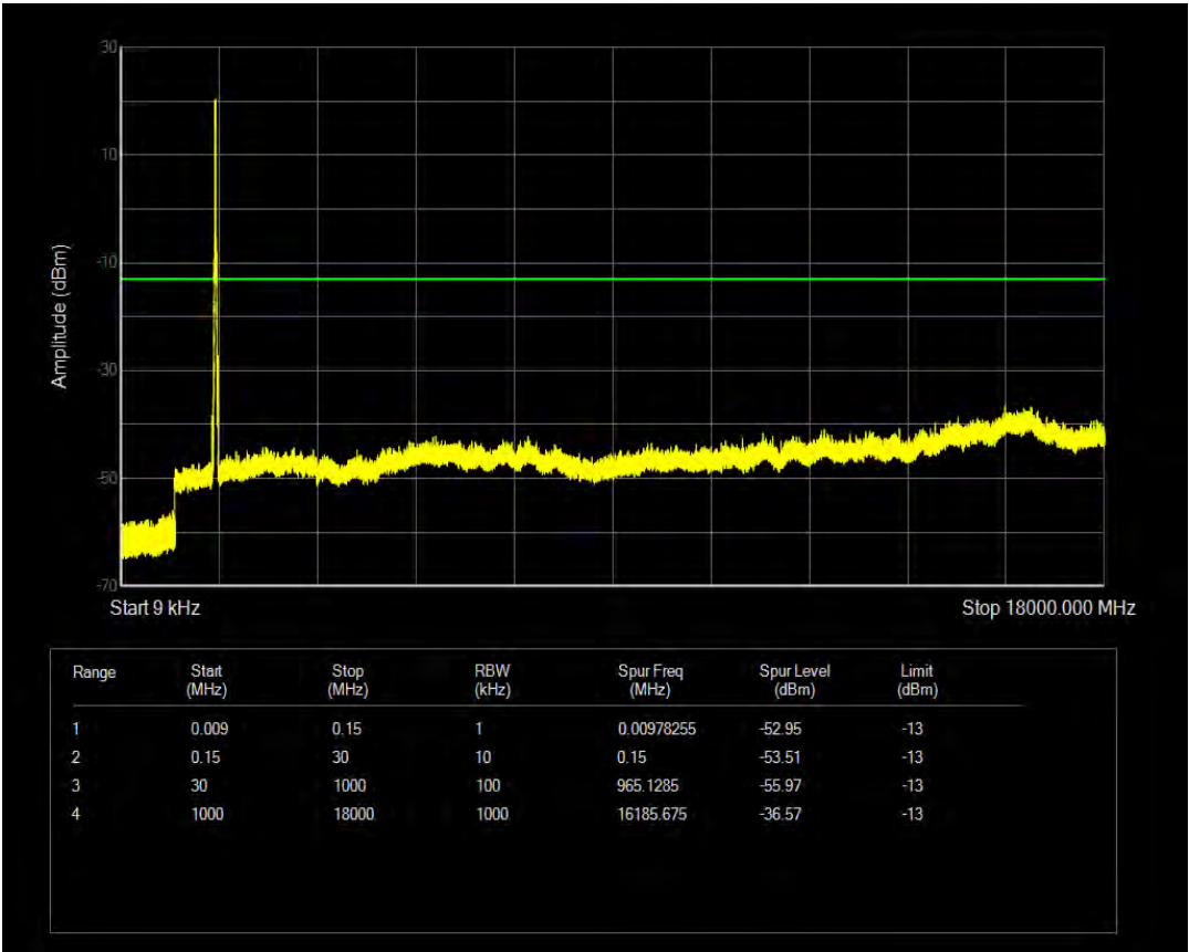
n66 SCS=15kHz CP QPSK BW=20MHz Channel=349000 RB=1@0
