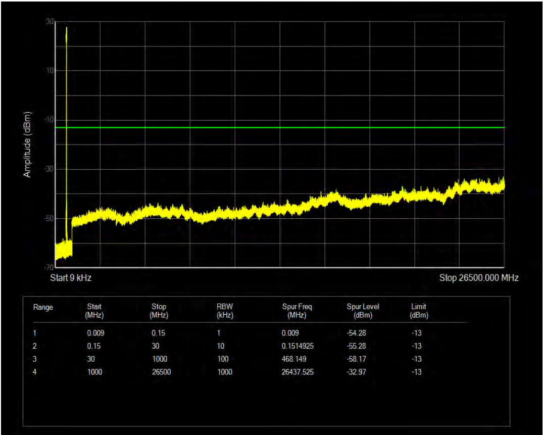
n71 SCS=15kHz CP QPSK BW=20MHz Channel=136100 RB=1@105
