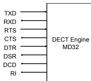
Fig. 2-3 V.24 Interface
