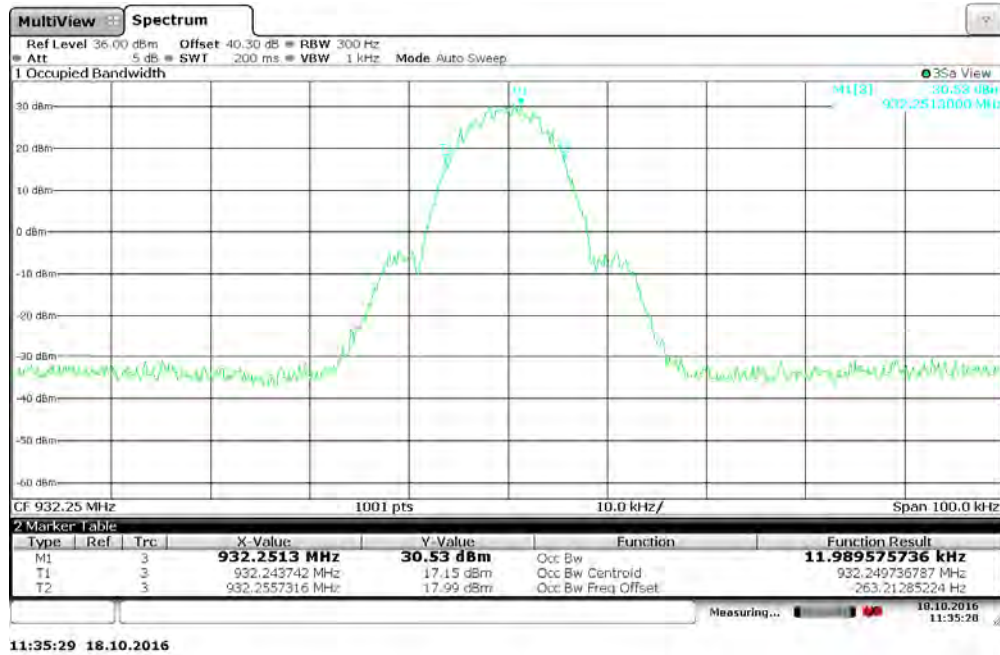
Figure 7.3.2-31: 932.25 MHz – 2FSK Mode
