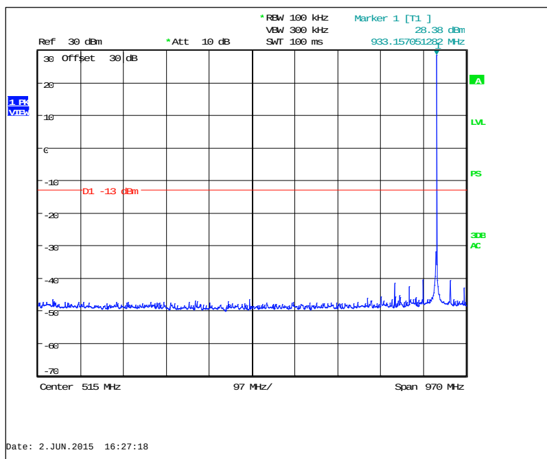
Figure 7.3.2-41: 932.25 MHz – 30MHz to 1GHz (Taitien TCXO)
