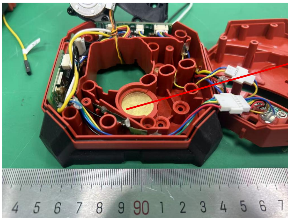
2.4 GHz Antenna
