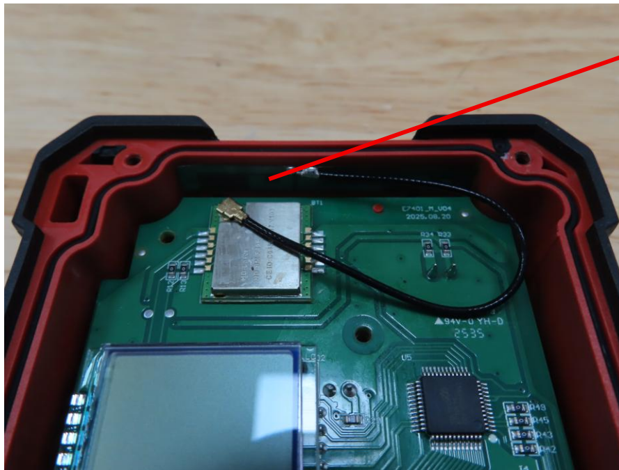
2.4 GHz Antenna
