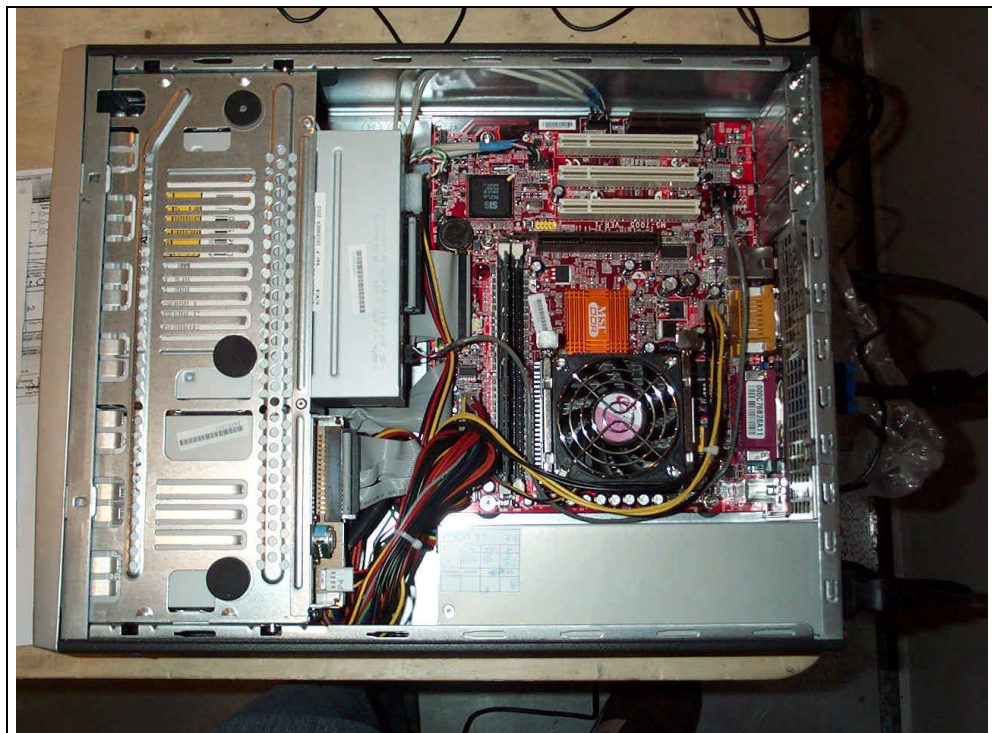
Bild 2. DUT, Innenansicht [DUT, inside]
