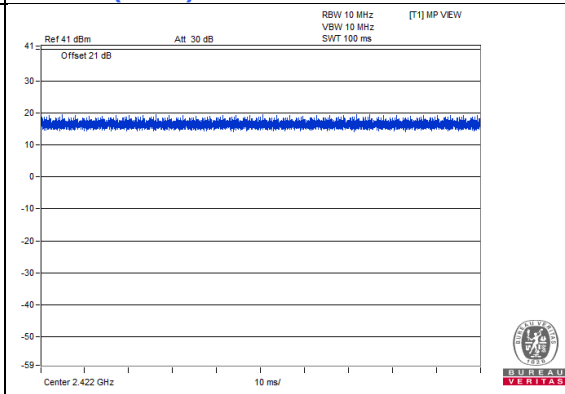
802.11n (HT40)
