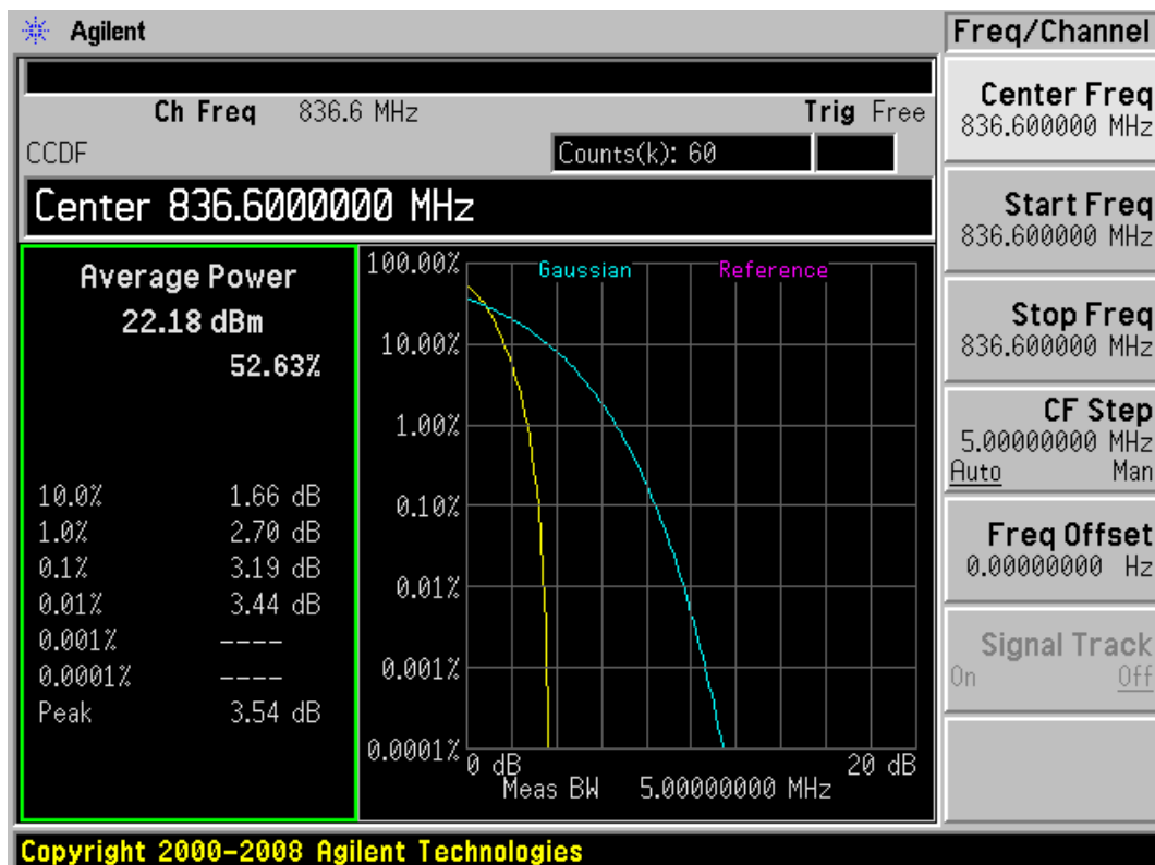
WCDMA Band V CH4183
