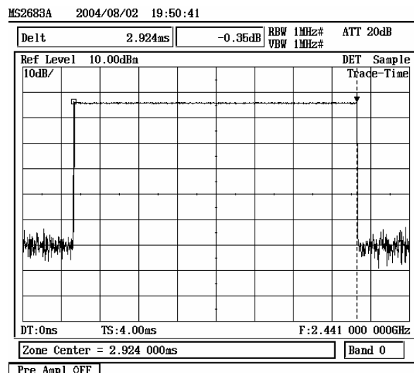
DH5 2441MHz
