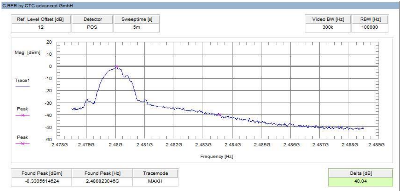
Plot 2: Upper band edge
