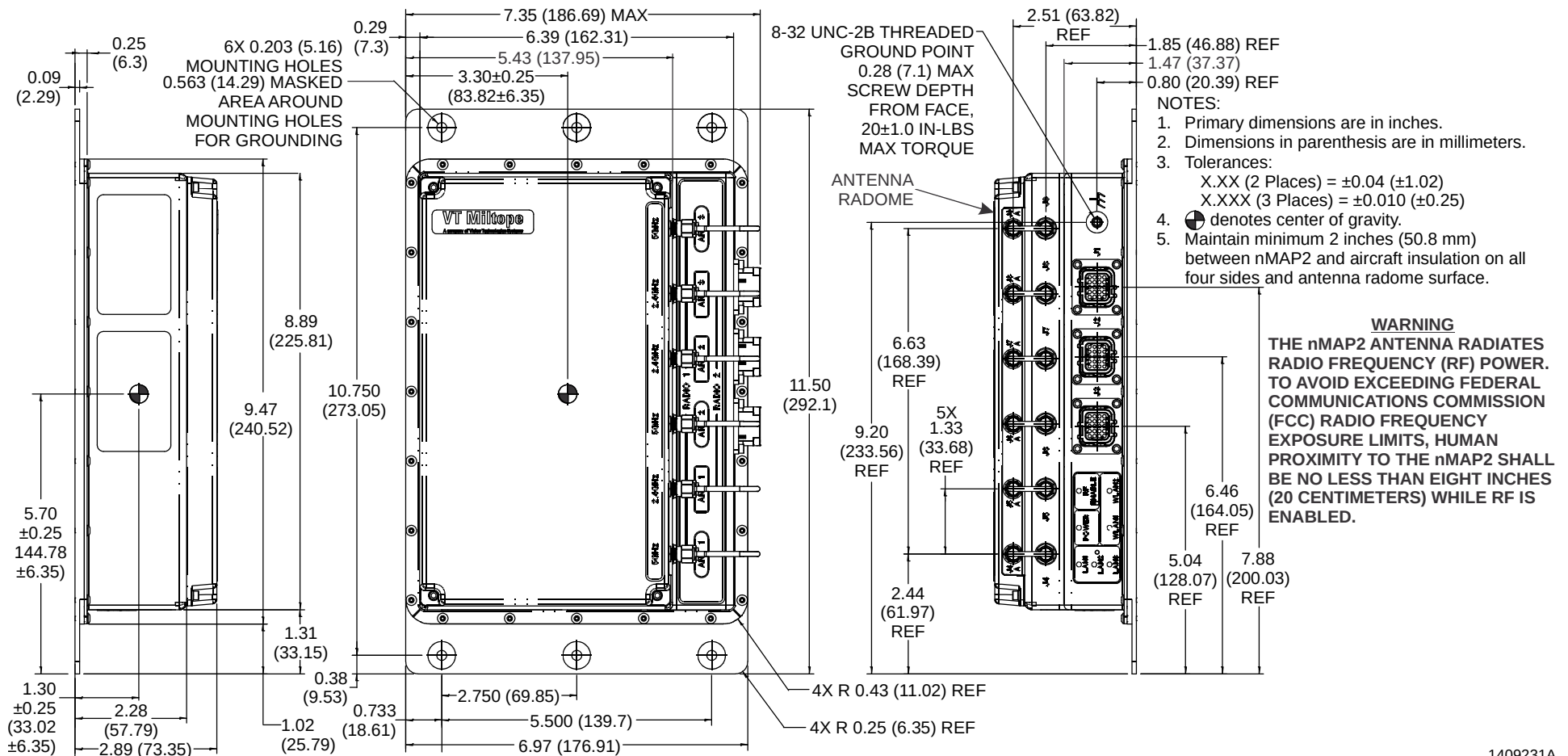
nMAP2 Access Point Outline Drawing
