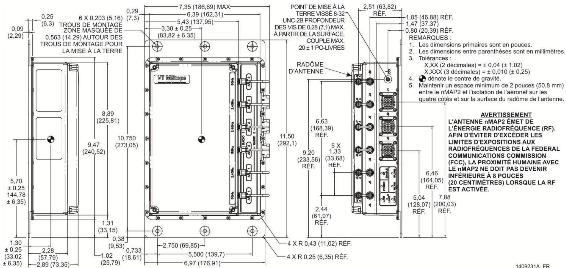
Schéma de point d'accès nMAP2
