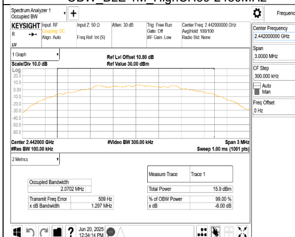
OBW_BLE 2M_MidCH20-2442MHz
